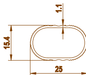
3254 0.167 kg/m
