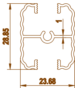
3247 0.404 kg/m
