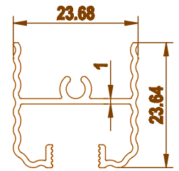
3246 0.319 kg/m
