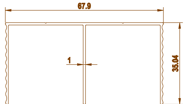
3249 0.526 kg/m
