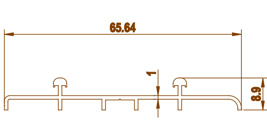
3225 0.280 kg/m
