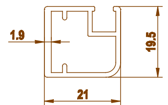
3252 0.328 kg/m
