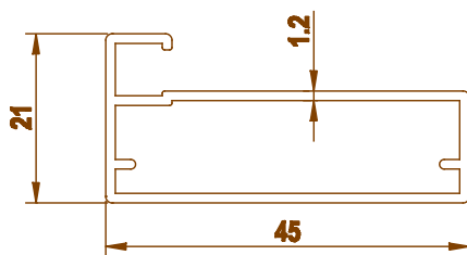
3250 0.431 kg/m
