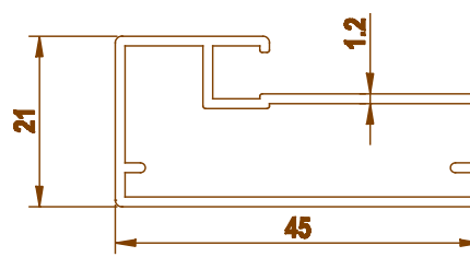
3251 0.456 kg/m
