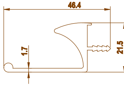
3241 0.574 kg/m
