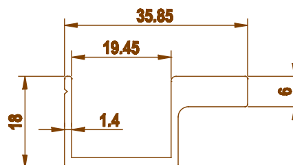
3719 0.478 kg/m
