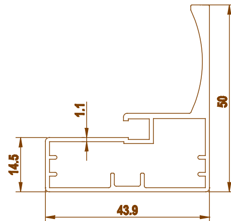
3715 0.725 kg/m
