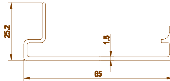
3604 0.465 kg/m
