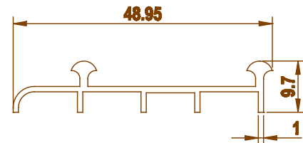
3702 0.252 kg/m
