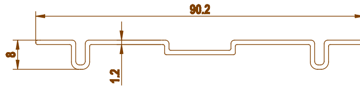
3603 0.400 kg/m
