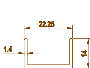
3718 0.218 kg/m
