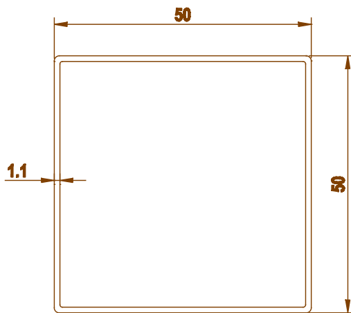
3706 0.592 kg/m
