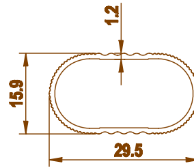
3511 0.198 kg/m
