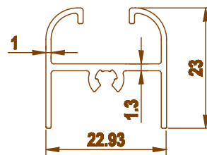
3516 0.263 kg/m
