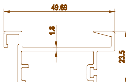
3541 0.514 kg/m
