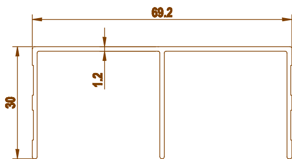
3513 0.494 kg/m
