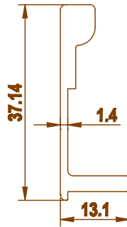
3510 0.369 kg/m
