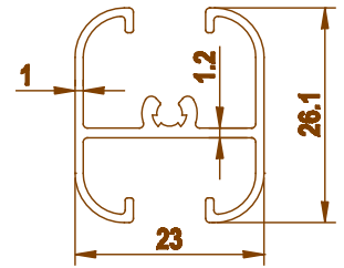
3512 0.308 kg/m
