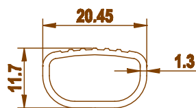
3537 0.172 kg/m
