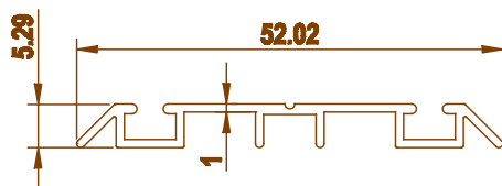
3515 0.242 kg/m
