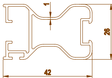
3296 0.495 kg/m
