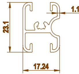
3288 0.283 kg/m
