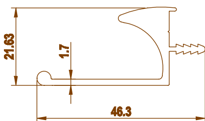
3298 0.537 kg/m
