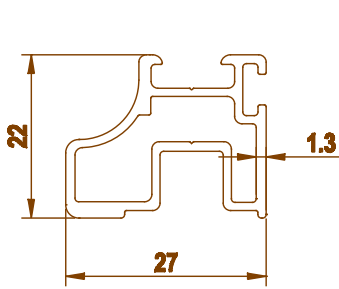
3287 0.394 kg/m
