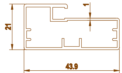
3297 0.443 kg/m
