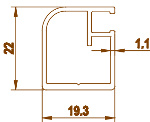
3295 0.284 kg/m
