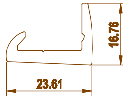
3292 0.339 kg/m
