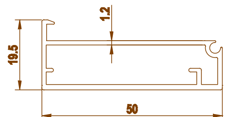
3300 0.495 kg/m
