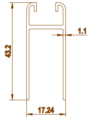
3290 0.354 kg/m
