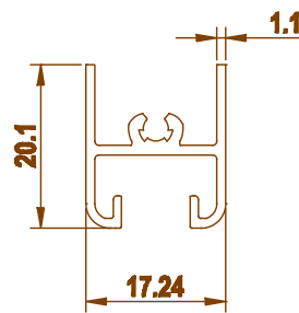
3289 0.234 kg/m
