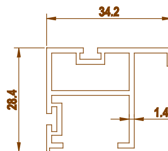
3708 0.502 kg/m
