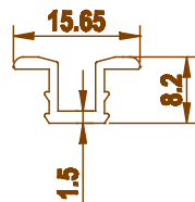
3528 0.102 kg/m
