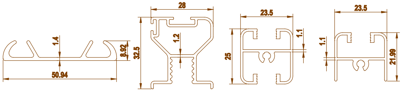
3522 0.364 kg/m
