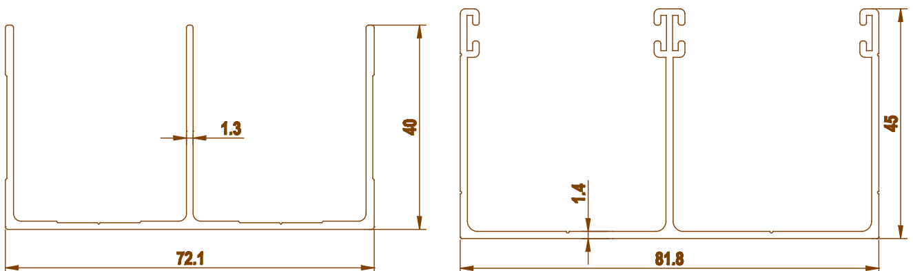
3533 0.724 kg/m
