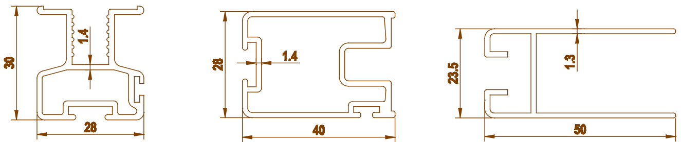
3530 0.544 kg/m
