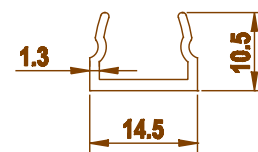
1998 0.118 kg/m
