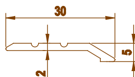
919 0.153 kg/m
