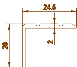
913 0.176 kg/m
