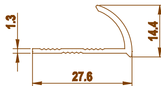
899 0.159 kg/m
