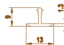
921 0.071 kg/m
