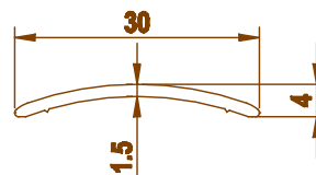
882 0.128 kg/m
