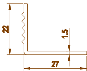
1125 0.207 kg/m
