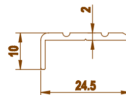
906 0.143 kg/m
