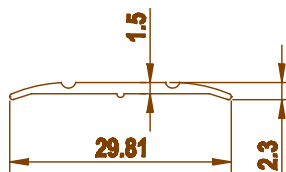
905 0.100 kg/m
