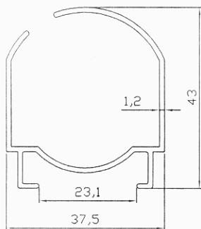
1151 0.461 kg/mt
