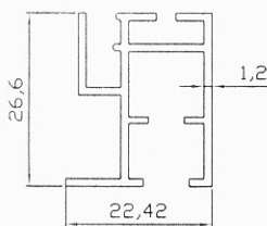
1204 0.355 kg/mt
