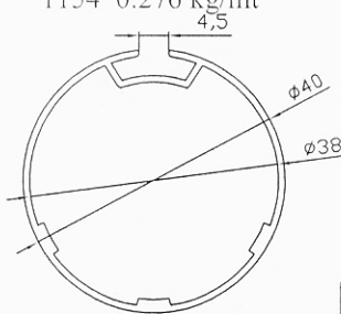
1181 0.407 kg/mt
