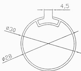
1180 0.278 kg/mt
