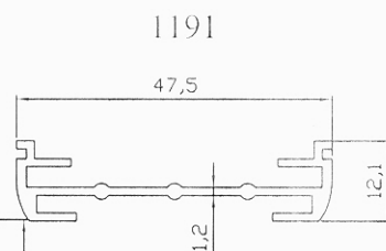
1191 0.359 kg/mt
