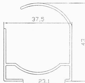
1218 0.459 kg/mt
