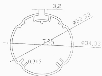
756 0.365 kg/mt
