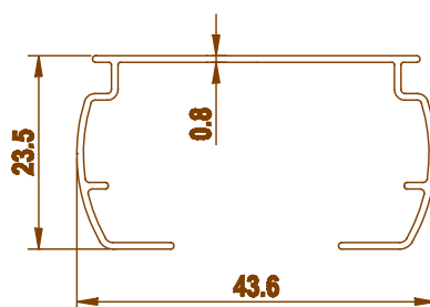
G397 0.243 kg/m
