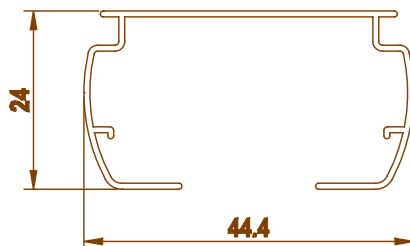
G139 0.256 kg/m
