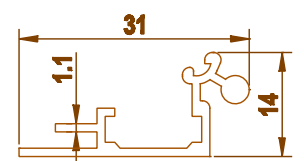
0000 0.215 kg/m
