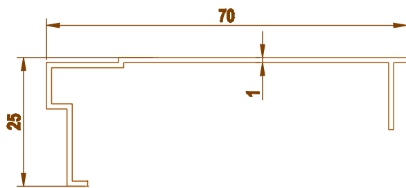
0000 0.308 kg/m
