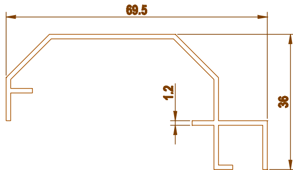
0000 0.405 kg/m
