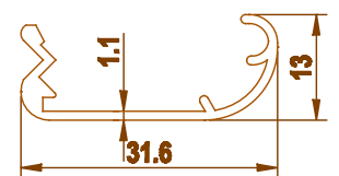
0000 0.197 kg/m
