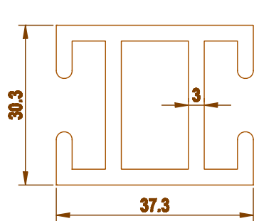
0000 1.222 kg/m
