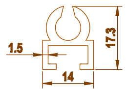
0000 0.259 kg/m
