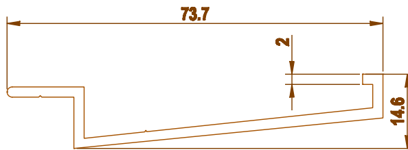
0000 0.499 kg/m
