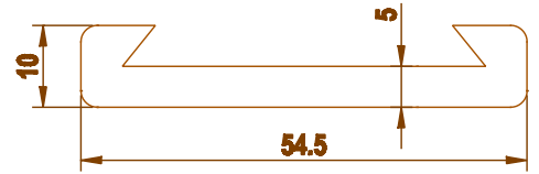
0000 0.397 kg/m
