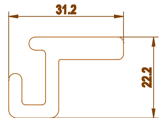
0000 0.732 kg/m
