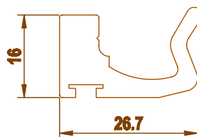
0000 0.665 kg/m
