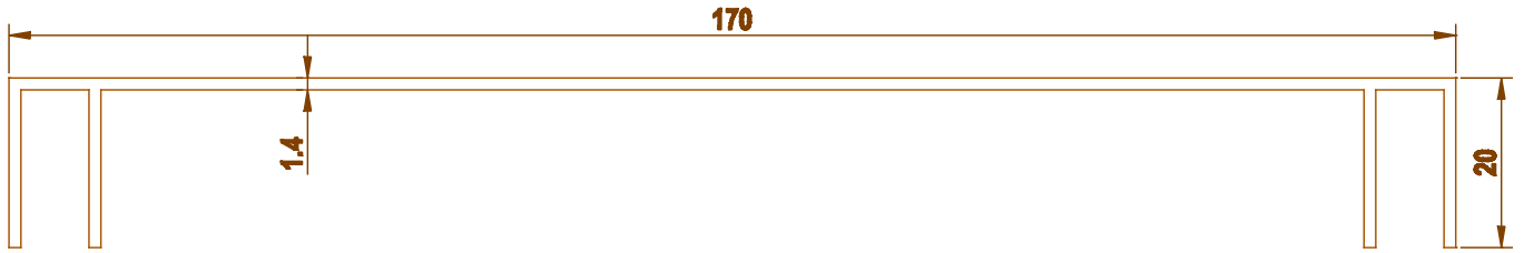
10093 0.927 kg/m
