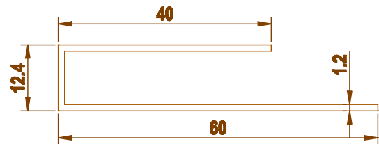
1506 0.357 kg/m
