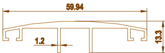
1497 0.471 kg/m
