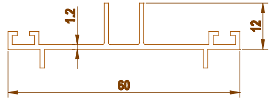
1496 0.347 kg/m
