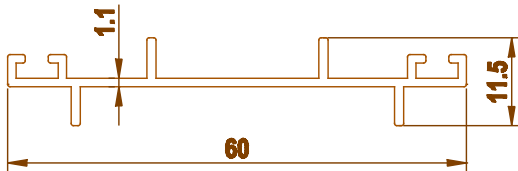
3144 0.297 kg/m
