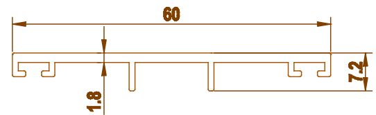
3145 0.372 kg/m
