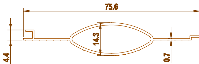
1554 0.301 kg/m
