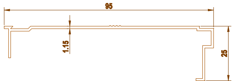
1565 0.428 kg/m
