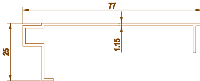
1551 0.378 kg/m
