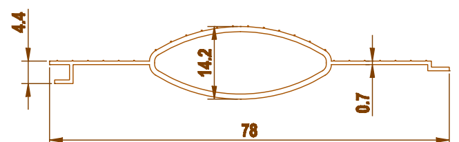
1601 0.303 kg/m
