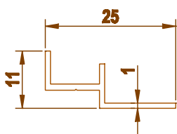
1564 0.111 kg/m
