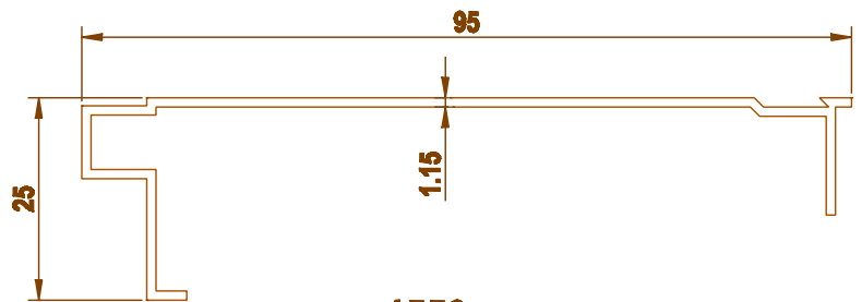
1550 0.445 kg/m
