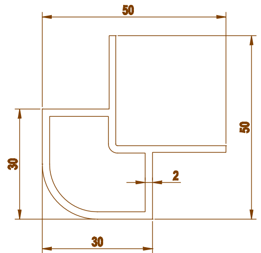
2065 0.763 kg/m
