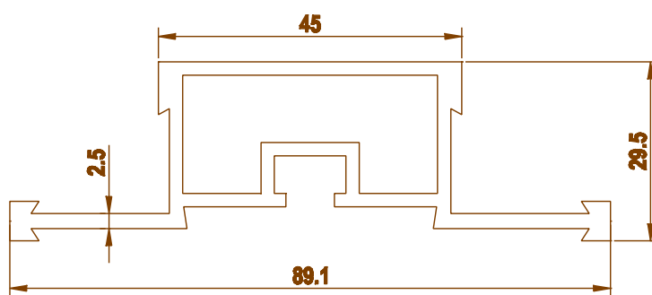
2413 1.486 kg/m
