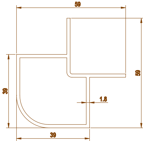
2064 0.887 kg/m
