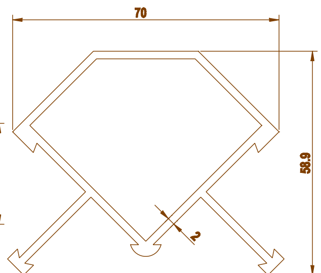
2414 1.409 kg/m
