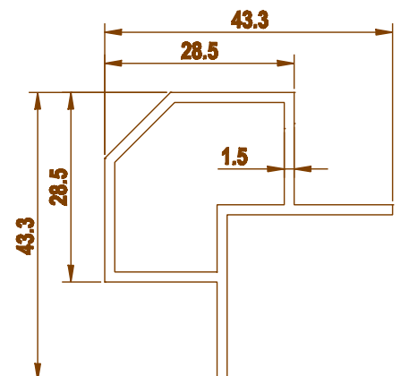
2299 0.536 kg/m
