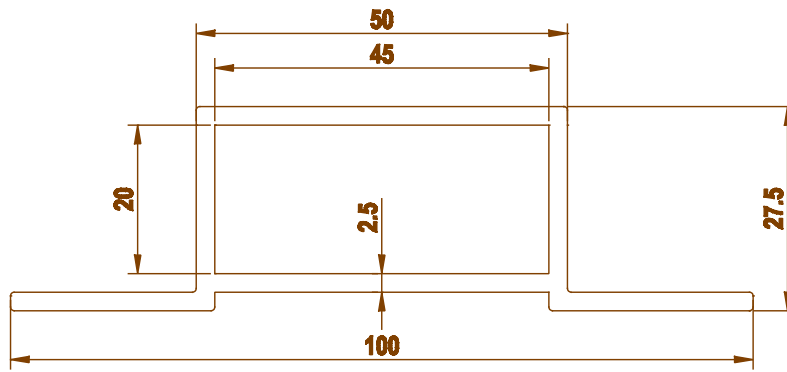
2084 1.315 kg/m
