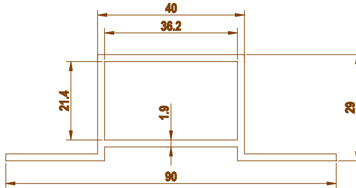
2074 0.928 kg/m
