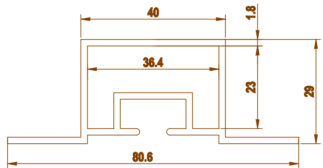
1936 0.970 kg/m
